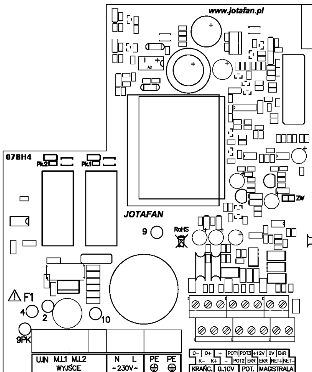
Rysunek 1 Schemat rozmieszczenia elementów na płycie INLET-010-2PK.
