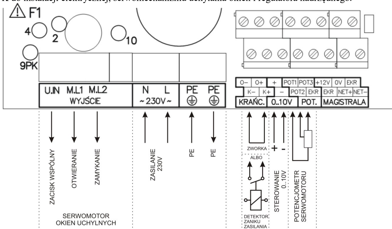
Rysunek 2 Opis zacisków regulatora wlotów INLET-010-2PK przy zadawaniu poziomu otwarcia okien napięciem analogowym 0 .. 10V i wyznaczania aktualnej pozycji okien za pomocą potencjometru serwomechanizmu.
