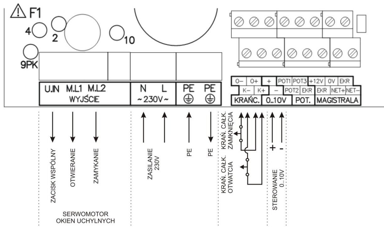
Rysunek 5 Opis zacisków regulatora wlotów INLET-010-2PK przy zadawaniu poziomu otwarcia okien napięciem analogowym 0 .. 10V i wyznaczania aktualnej pozycji okien za pomocą pomiaru czasu przejazdu pomiędzy krańcówkami 0% i 100%.
