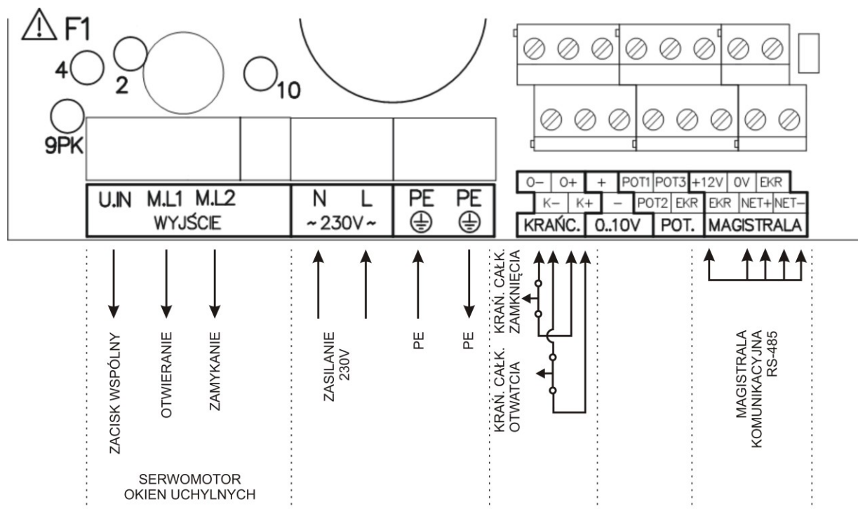
Rysunek 4 Opis zacisków regulatora wlotów INLET-010-2PK przy zadawaniu poziomu otwarcia okien za pomocą interfejsu RS-485 i wyznaczania aktualnej pozycji okien za pomocą pomiaru czasu przejazdu pomiędzy krańcówkami 0% i 100%.
