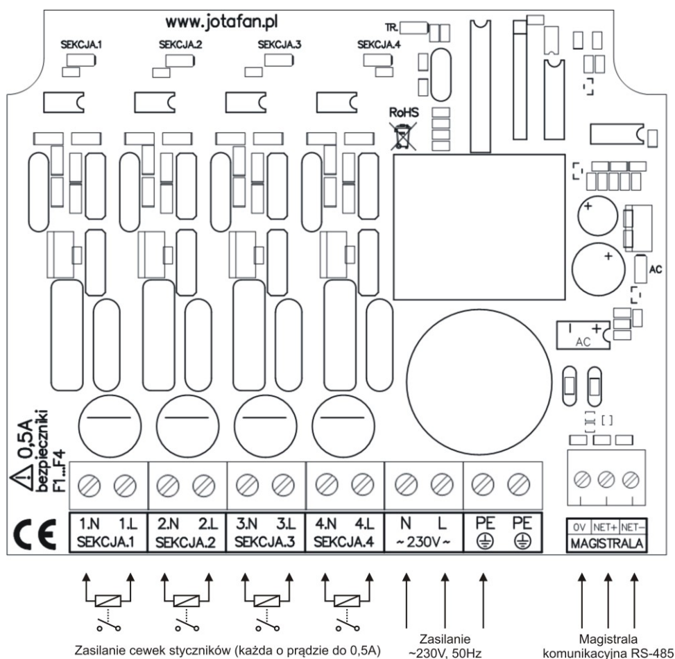
Rysunek 1 Opis wyprowadzeń modułu 4ZW
