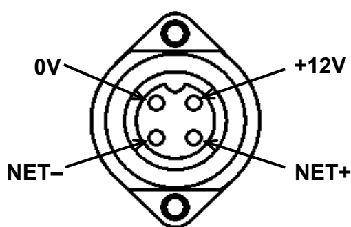
Rysunek 1 Rozmieszczenie zacisków w gnieździe przyłączeniowym
