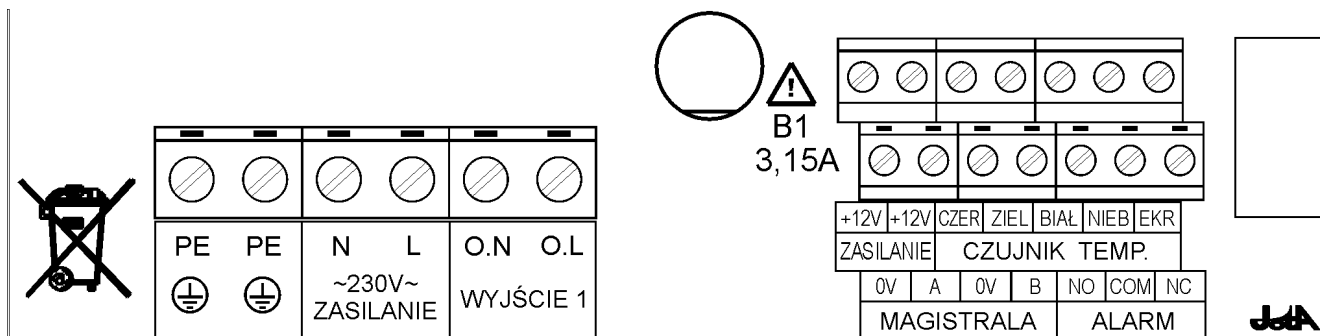
Rys. 1: Rozmieszczenie zacisków połączeniowych regulatora TERMISTAT-AL-010-LCD
