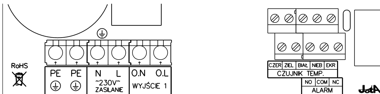
Rys. 1: Rozmieszczenie zacisków połączeniowych regulatora TERMISTAT-6-AL-LCD
