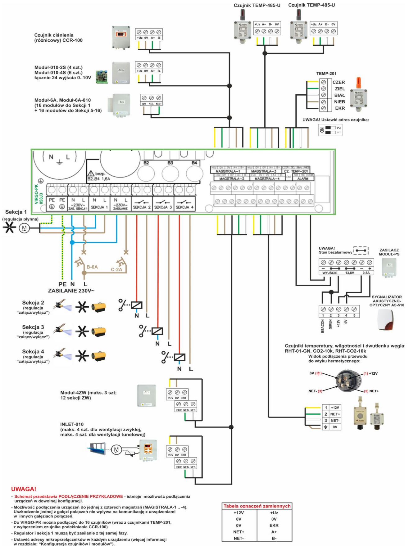
Rys. 2. Schemat przykładowego połączenia regulatora z zasilaniem, odbiornikami, czujnikami i modułami rozszerzeń.
