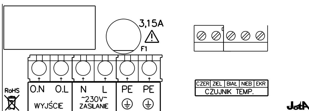
Rysunek 1 Rozmieszczenie zacisków połączeniowych regulatora TERMISTAT-3
