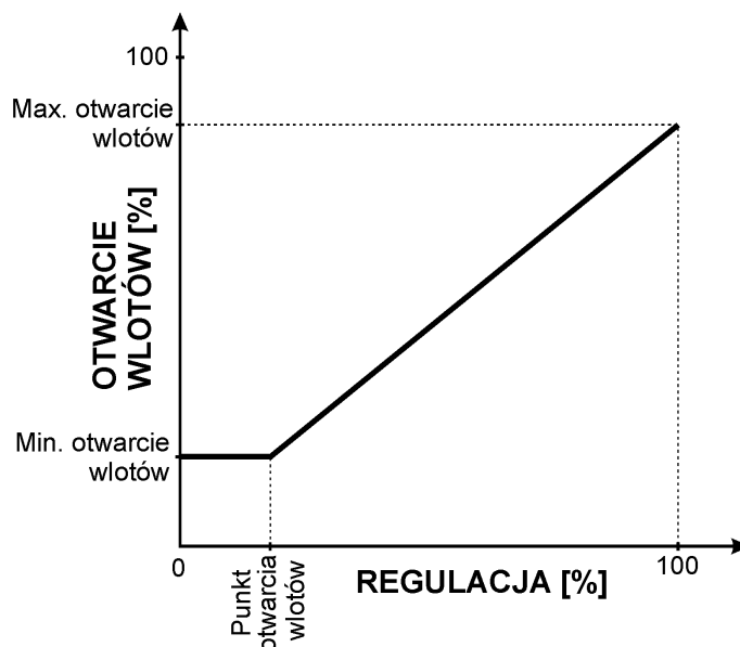
Rysunek 3. Wpływ zmian poziomu regulacji na analogowe napięcie wyjściowe.
