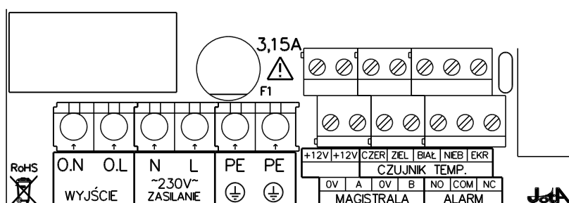
Rysunek 1 Rozmieszczenie zacisków połączeniowych regulatora TERMISTAT-3-AL-010
