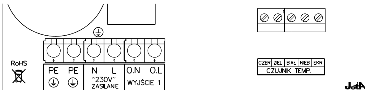
Rysunek 1 Rozmieszczenie zacisków połączeniowych regulatora TERMISTAT-6
