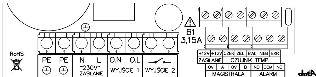
Rys. 1: Rozmieszczenie zacisków połączeniowych regulatora TERMISTAT-6-2S-485
