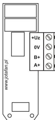
Rys. 3. Rozmieszczenie zacisków połączeniowych interfejsu RS-485 do komunikacji z PC
