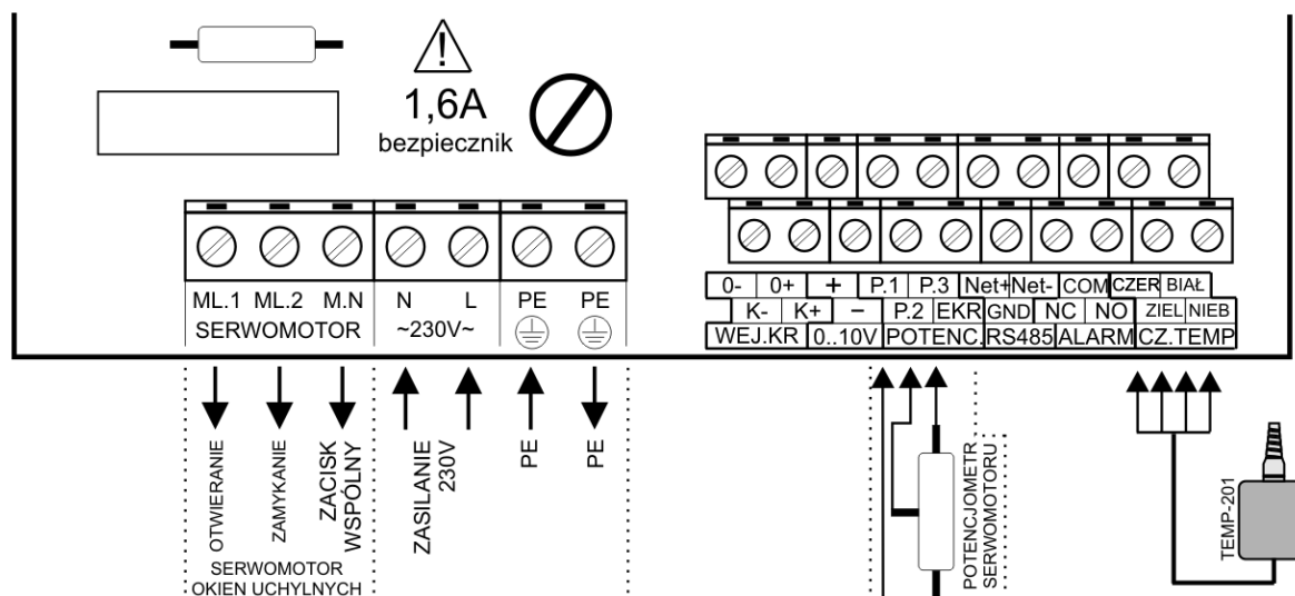
Rysunek 1 Opis zacisków regulatora wlotów TERMISTAT-INL przy wyznaczaniu aktualnej pozycji okien za pomocą potencjometru serwomotoru.
