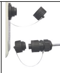
Schemat podłączenia modułu szalki z wtykiem hermetycznym.
