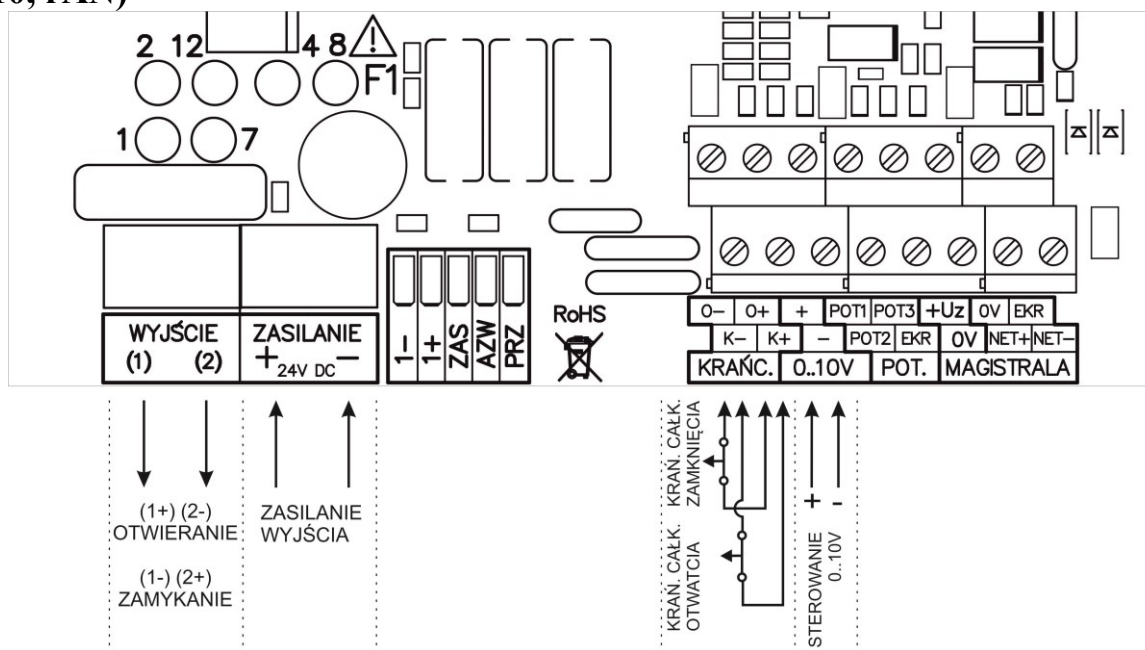
Rysunek 1 Opis zacisków regulatora wlotów INLET-010-LIN przy zadawaniu poziomu otwarcia okien napięciem analogowym 0 .. 10V i wyznaczania aktualnej pozycji okien za pomocą pomiaru czasu przejazdu pomiędzy krańcówkami 0% i 100%.
