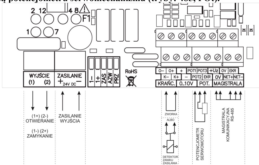
Rysunek 1 Opis zacisków regulatora wlotów INLET-010-LIN przy zadawaniu poziomu otwarcia okien za pomocą interfejsu RS-485 i wyznaczania aktualnej pozycji okien za pomocą potencjometru serwomechanizmu.
