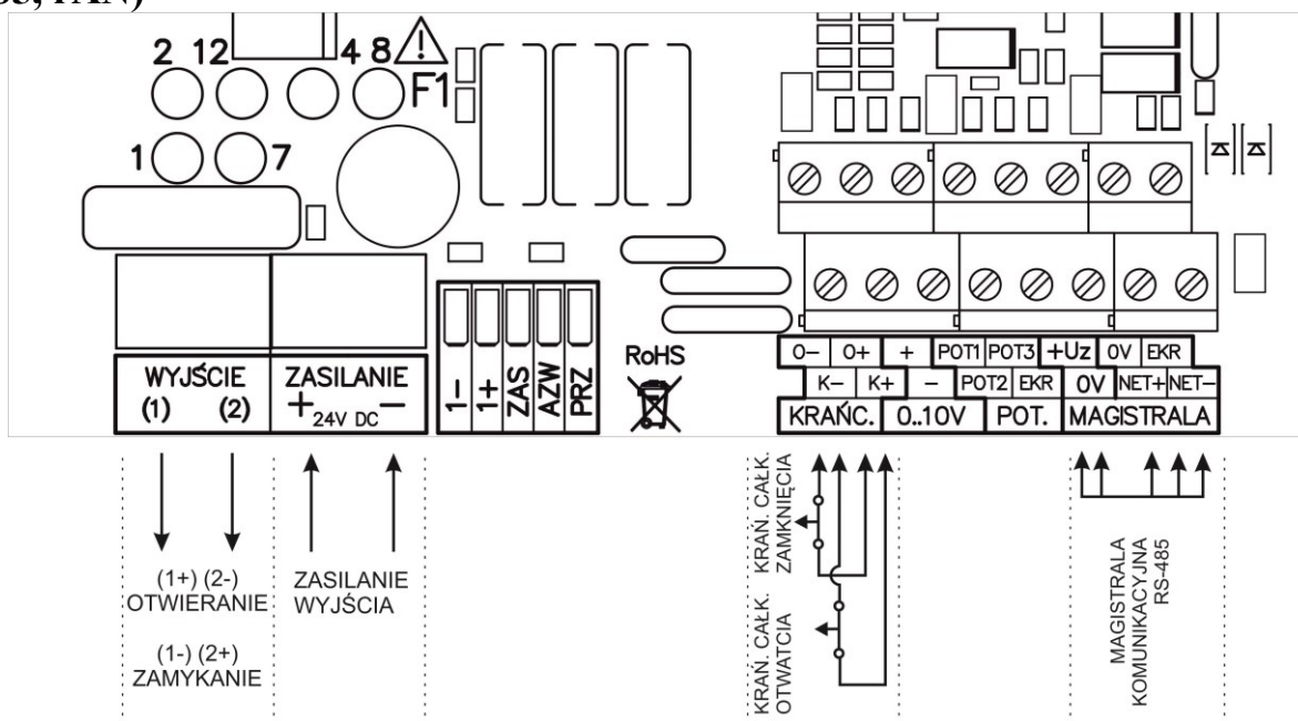
Rysunek 1 Opis zacisków regulatora wlotów INLET-010-LIN przy zadawaniu poziomu otwarcia okien za pomocą interfejsu RS-485 i wyznaczania aktualnej pozycji okien za pomocą pomiaru czasu przejazdu pomiędzy krańcówkami 0% i 100%.
