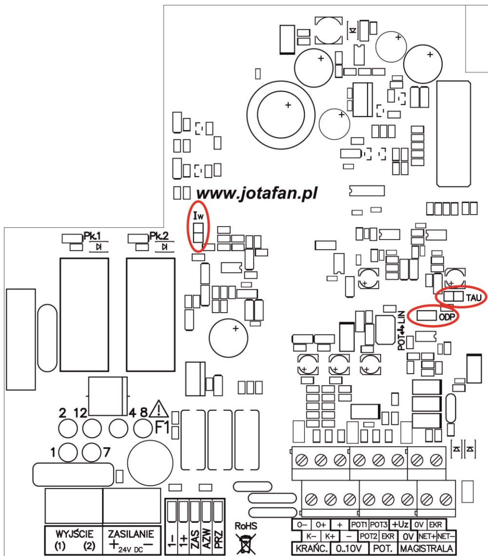
Rysunek 1 Schemat rozmieszczenia elementów na płycie INLET-010-LIN dla wersji PCB 078J3.
