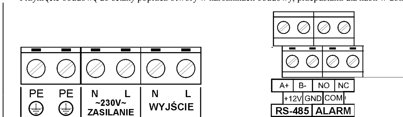
Rys. 1: Rozmieszczenie zacisków połączeniowych regulatora MIREF-6-AL-485
