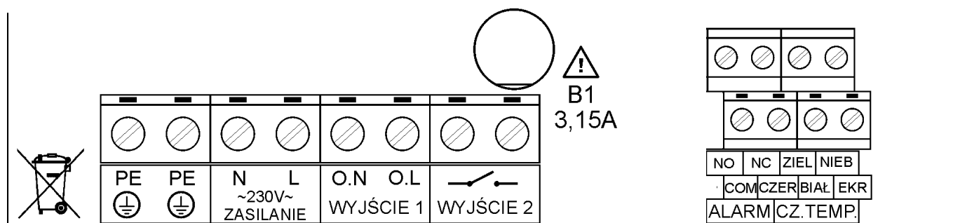
Rys. 1: Rozmieszczenie zacisków połączeniowych regulatora TERMISTAT-LCD
