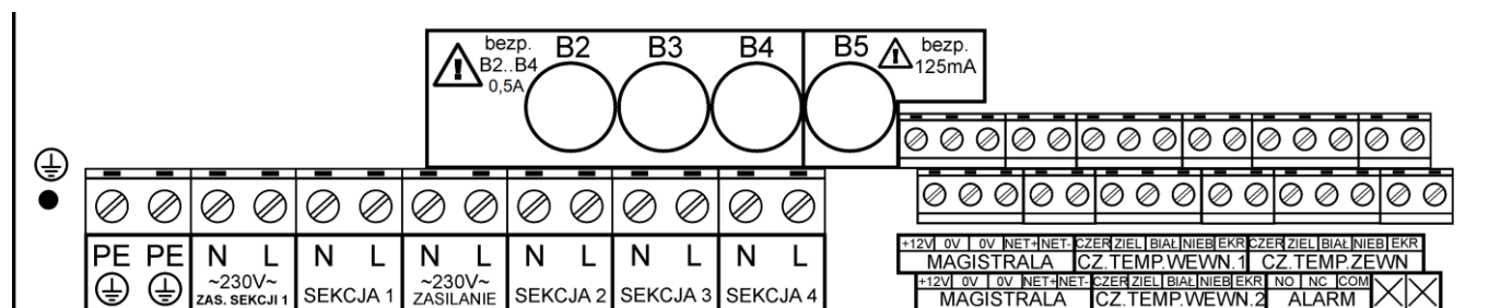
Rys. 1: Rozmieszczenie zacisków połączeniowych regulatora BITERMO-4S-485-LCD
