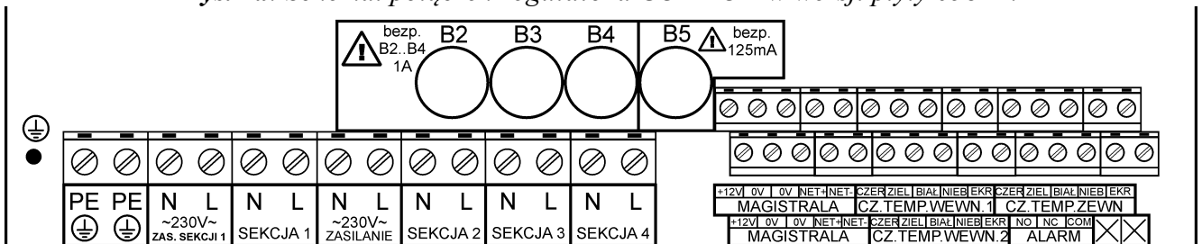
Rys. 1b: Opis listew zaciskowych regulatora COMBO+ w wersji płyty 058G2.
