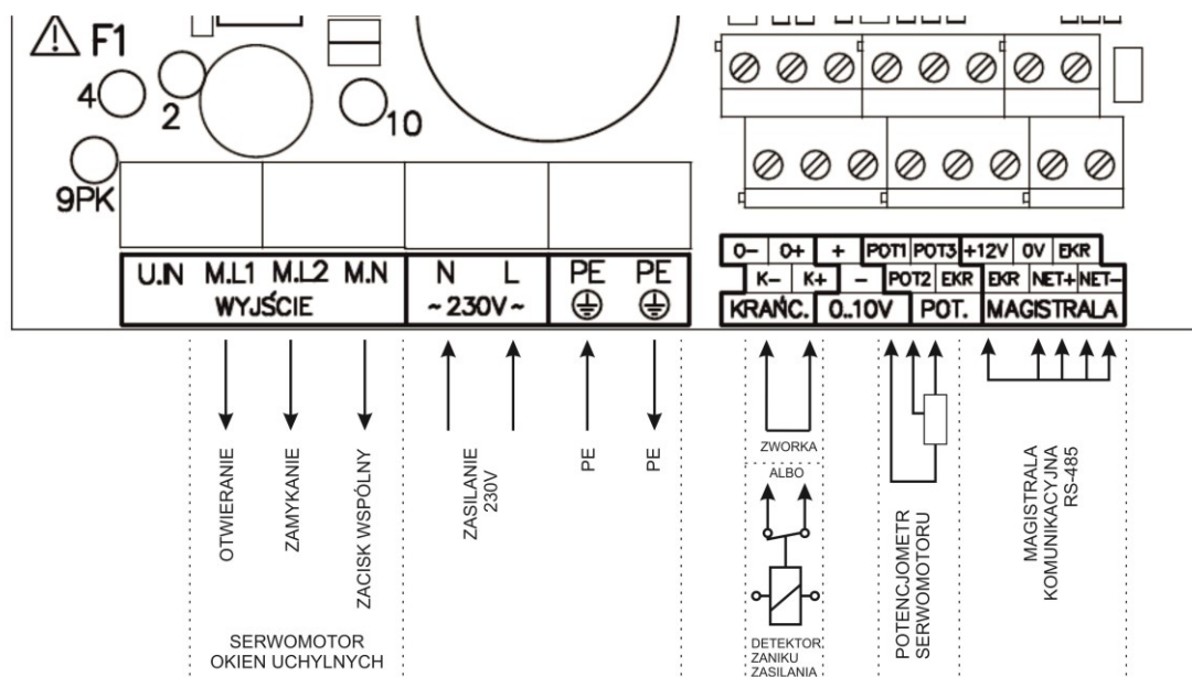
Rysunek 1 Opis zacisków regulatora wlotów INLET-010 przy zadawaniu poziomu otwarcia okien za pomocą interfejsu RS-485 i wyznaczania aktualnej pozycji okien za pomocą potencjometru serwomechanizmu.
