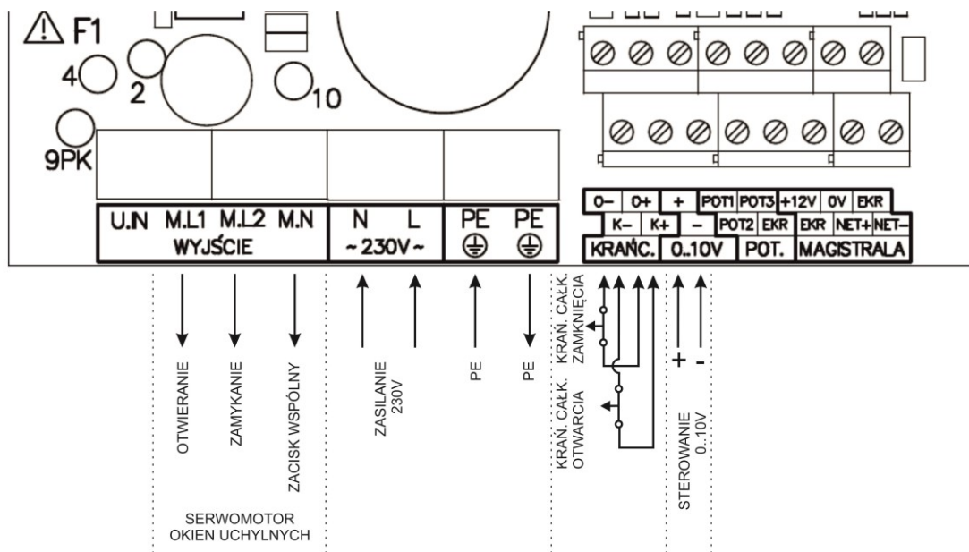
Rysunek 1 Opis zacisków regulatora wlotów INLET-010 przy zadawaniu poziomu otwarcia okien napięciem analogowym 0 .. 10V i wyznaczania aktualnej pozycji okien za pomocą pomiaru czasu przejazdu pomiędzy krańcówkami 0% i 100%.
