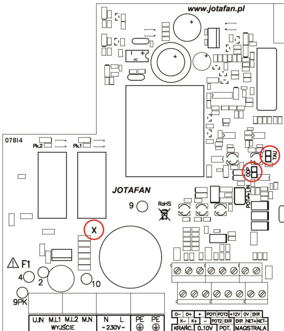
Rysunek 1 Schemat rozmieszczenia elementów na płycie INLET-010 dla wersji PCB 07814.
