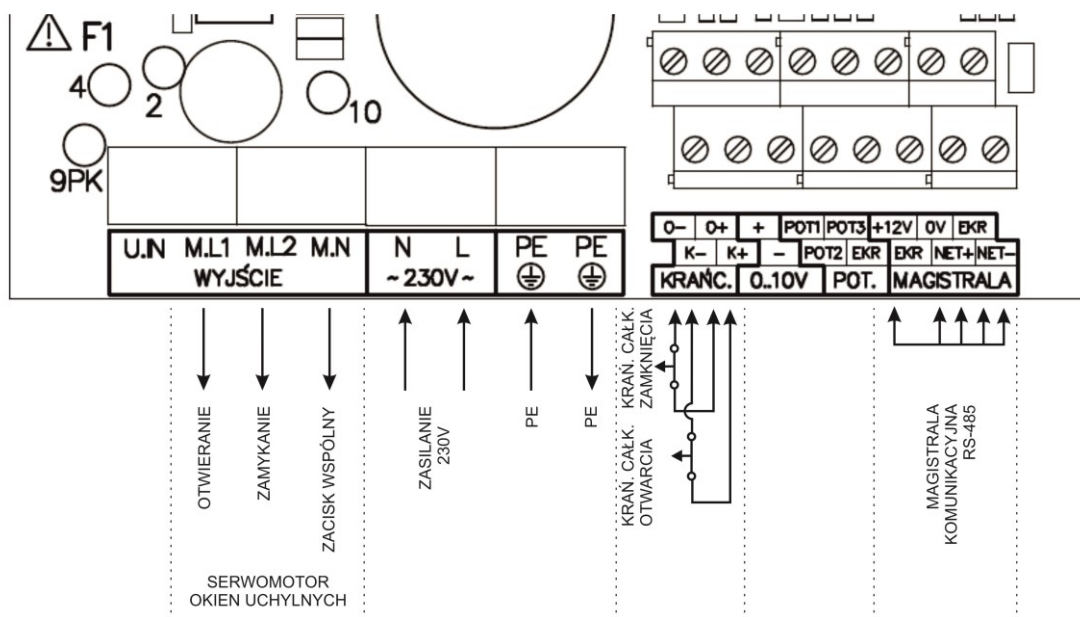
Rysunek 1 Opis zacisków regulatora wlotów INLET-010 przy zadawaniu poziomu otwarcia okien za pomocą interfejsu RS-485 i wyznaczania aktualnej pozycji okien za pomocą pomiaru czasu przejazdu pomiędzy krańcówkami 0% i 100%.
