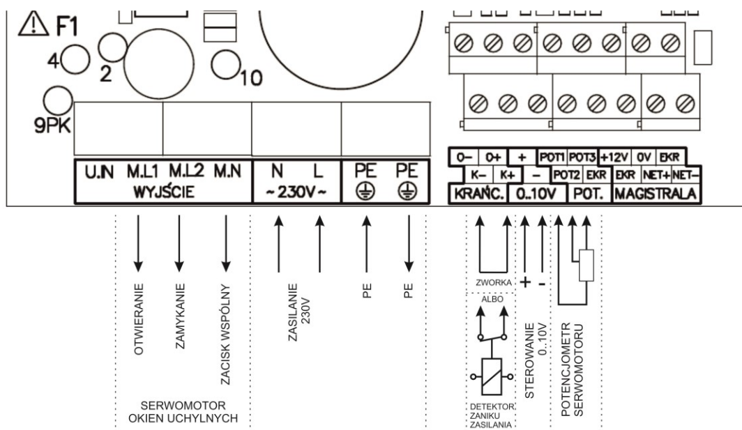
Rysunek 1 Opis zacisków regulatora wlotów INLET-010 przy zadawaniu poziomu otwarcia okien napięciem analogowym 0 .. 10V i wyznaczania aktualnej pozycji okien za pomocą potencjometru serwomechanizmu.
