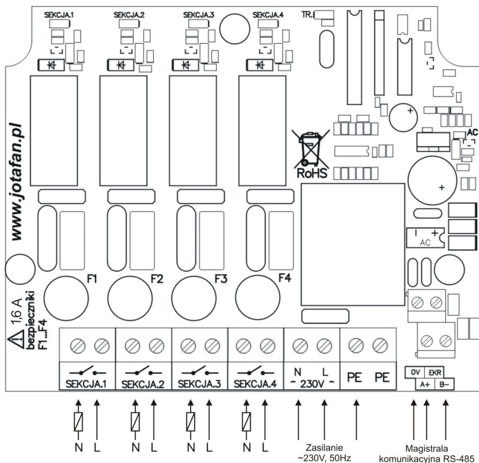
Rysunek 1 Opis wyprowadzeń modułu 4ZW-PK
