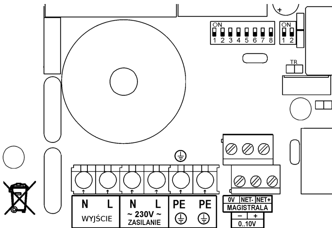
Rys. 1 Modułu 6A-010-LED-AR - widok wyprowadzeń na płycie wewnątrz obudowy
