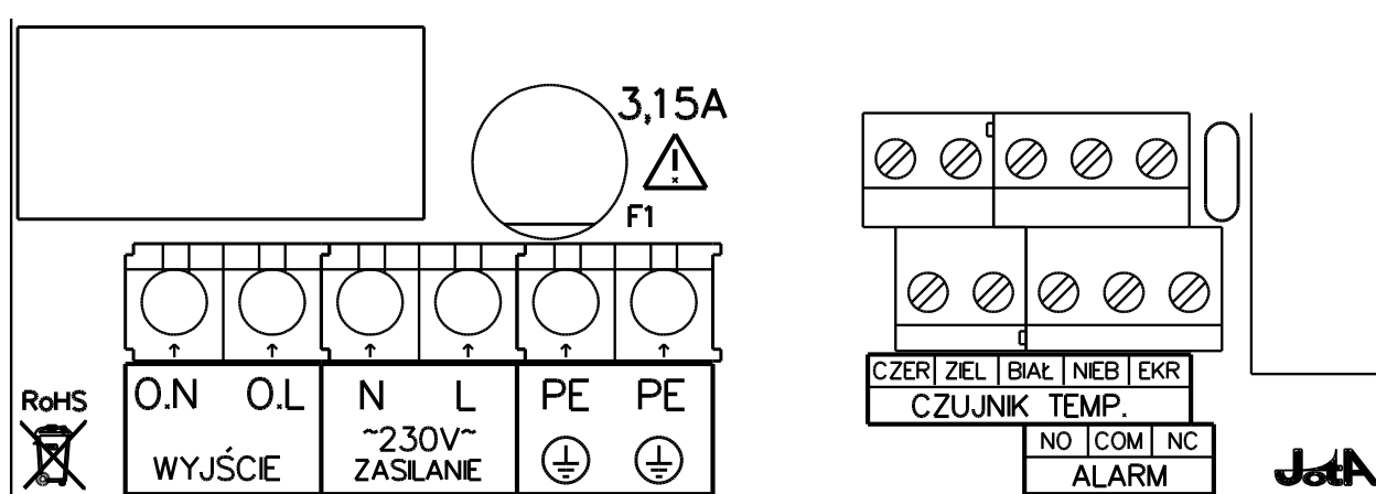
Rysunek 1 Rozmieszczenie zacisków połączeniowych regulatora TERMISTAT-3-AL
