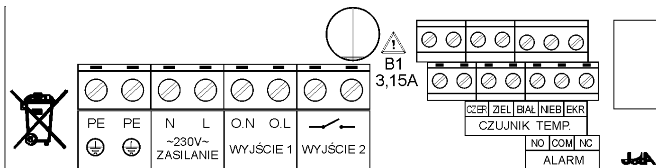
Rys. 1: Rozmieszczenie zacisków połączeniowych regulatora TERMISTAT-6-2S-LCD
